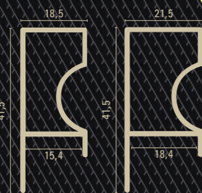
Perfil para Vidro V03
