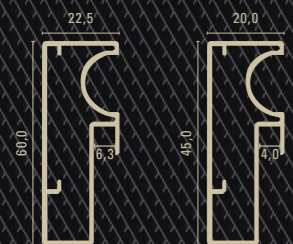
Perfil para Vidro V03
